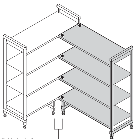
Unidade de Canto Unidade Inicial + Add-On usando 1 jogo de Conectores de Canto por prateleira e 2 Armações.
