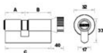
Llave de puntos de 6 claves 6 pins flat key Chave de pontos de 6 pinos
