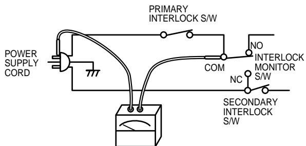
(ohmmeter) – Fig. b –
