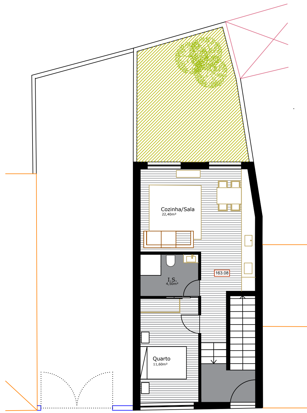
Planta R/C
