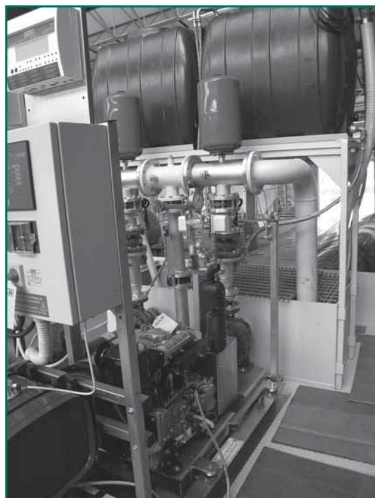
Vano pompe con gruppo antincendio montato.
