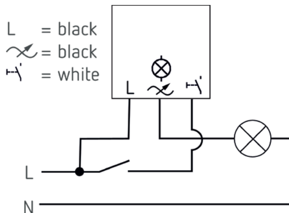
Figura 3. Com ligações simples a 3 fios adapta-se a qualquer circuito, sem necessitar de neutro.
