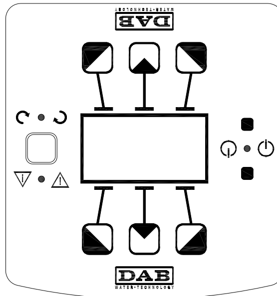
Fig. 7: Kontrollpanel
