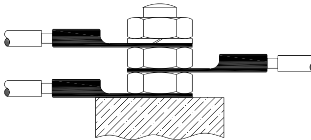
Resim 2: Toprak bağlantısı
