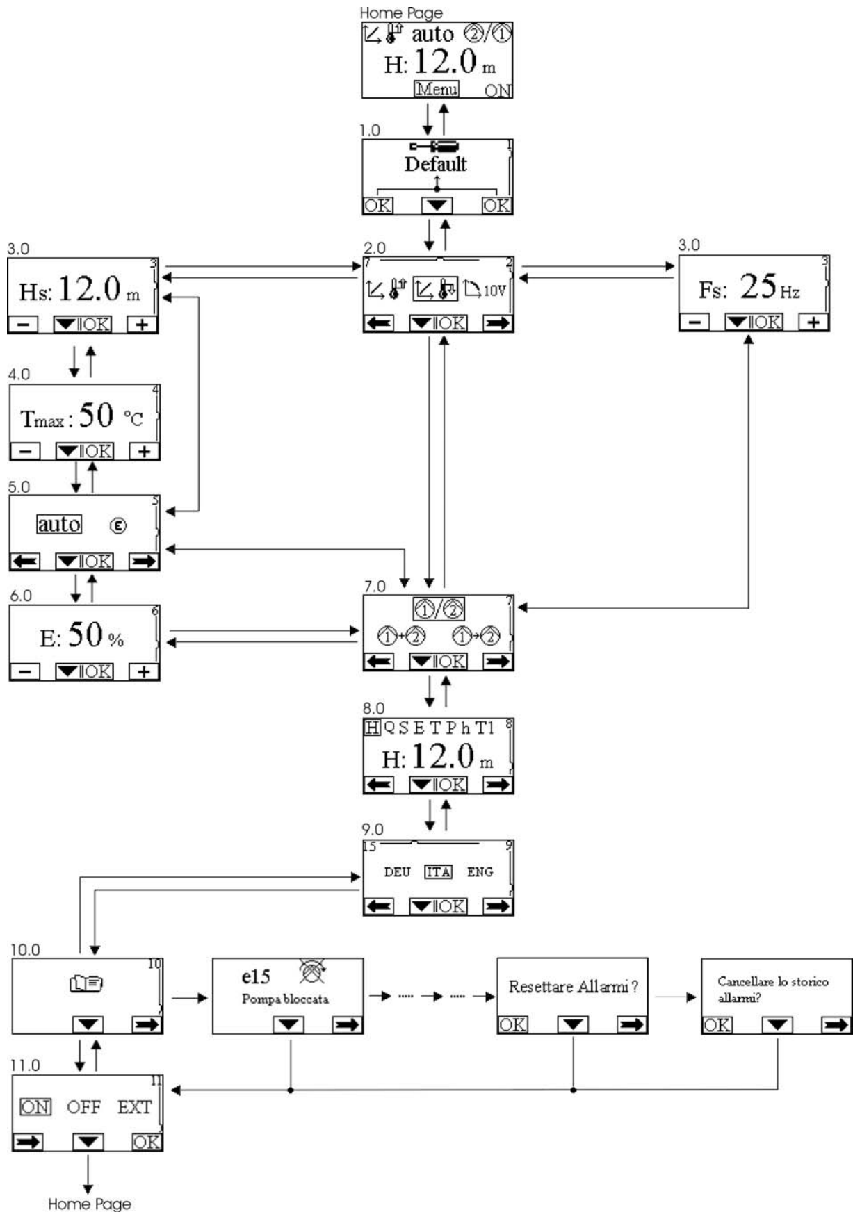
Σχήμα 8: Μενού MCE
