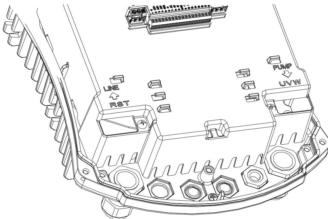
Figura 1: Conexiuni Electrice
