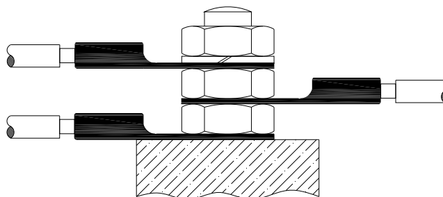
Slika 2: Ozemljitev
