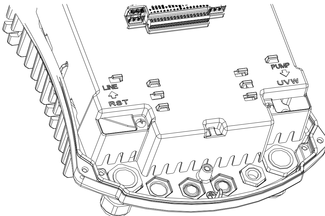
Σχήμα 1: Ηλεκτρική Συνδεσμολογία
