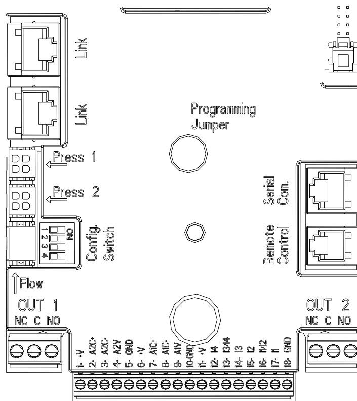
Slika 3: Priključki
