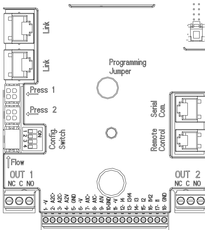
Figura 3: Conexiones
