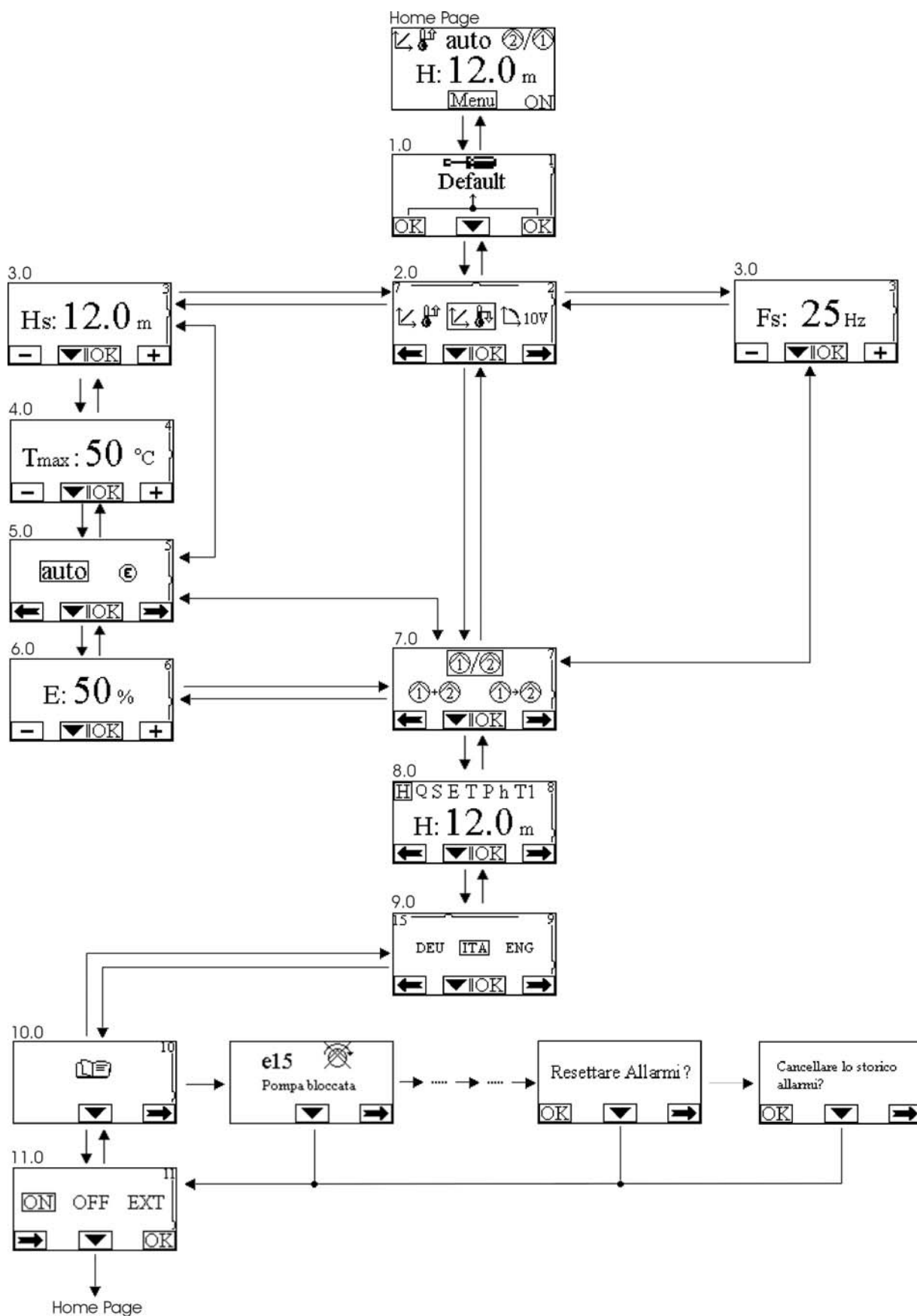
Figura 8: Meniu MCE
