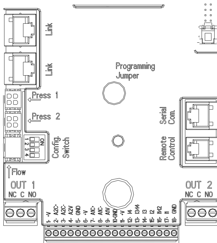
Figura 3: Conexiuni
