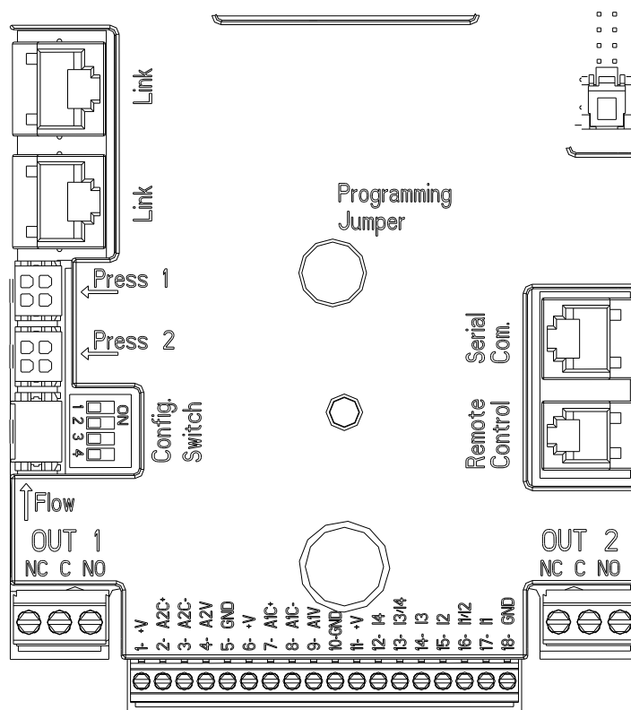
Схема 3: Соединения
