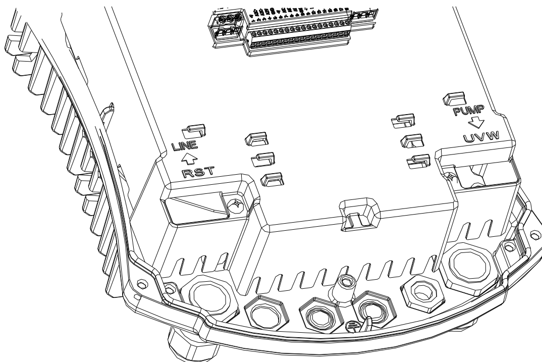
Figura 1: Conexiones eléctricas
