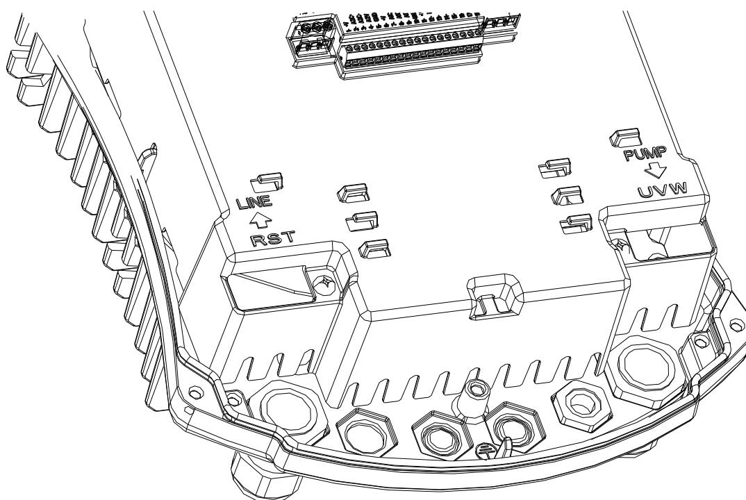
Figure 1: Connexions électriques
