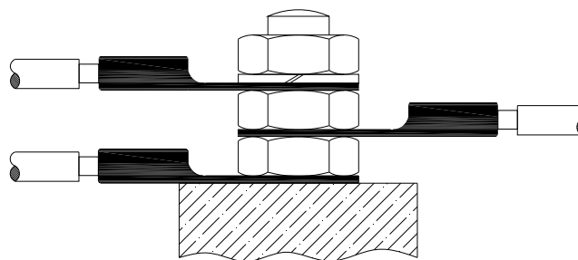
Fig 2: Jordanslutning
