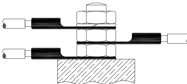
Abbildung 2: Erdungsanschluss
