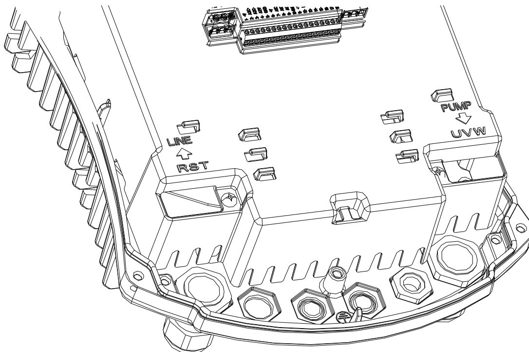
Figura 1: Connessioni Elettriche
