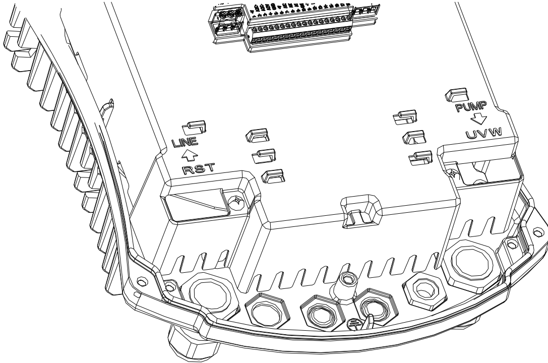
Resim 1: Elektrik Bağlantıları
