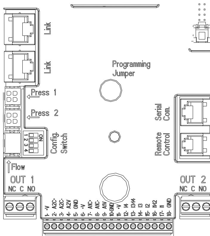
Fig. 3: Anslutningar
