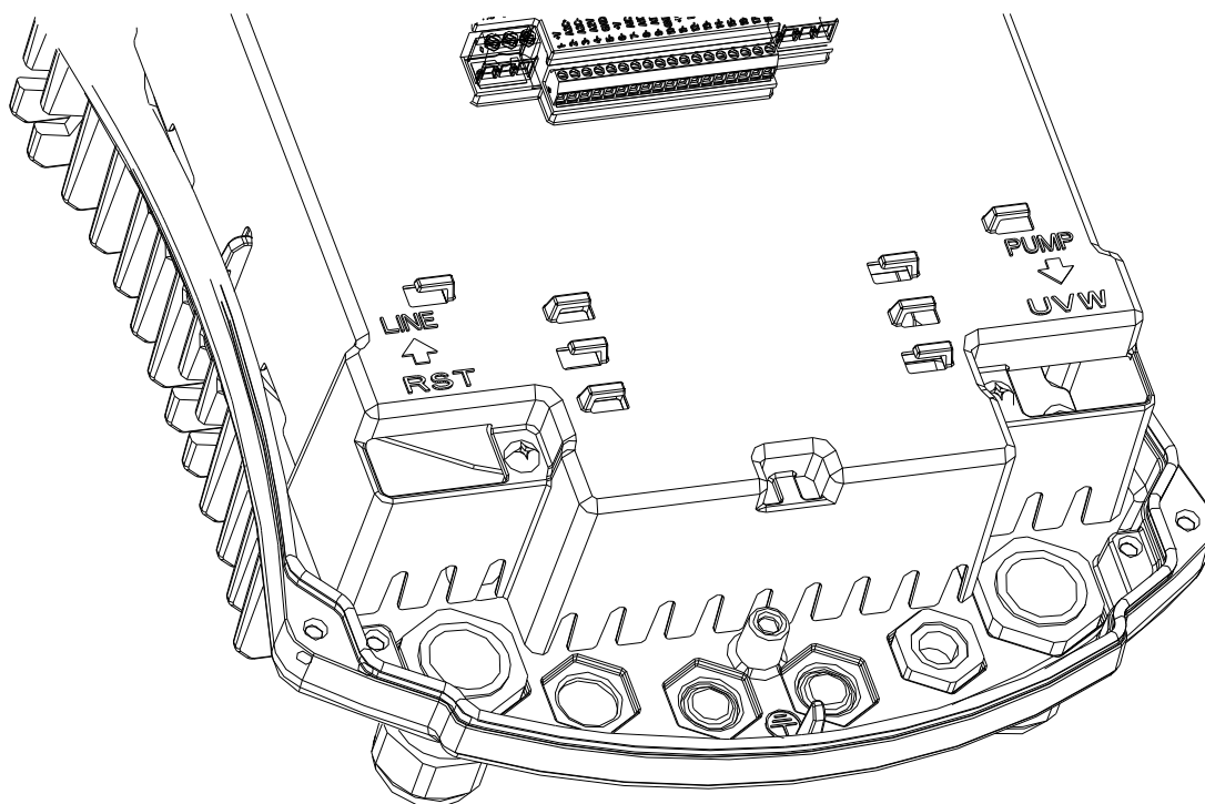
Slika 1: Električni priključki
