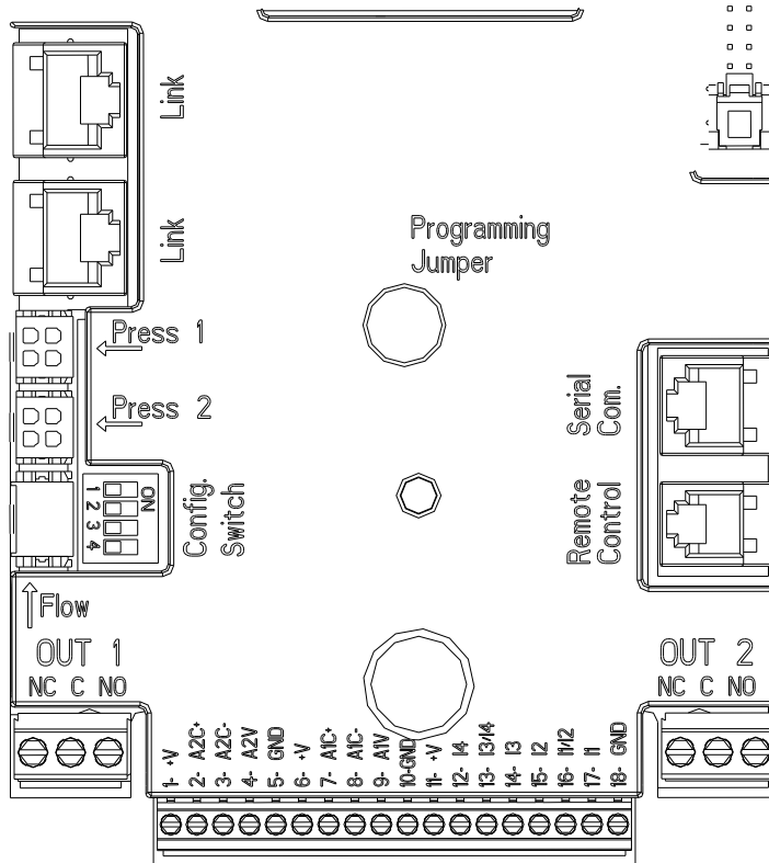
Resim 3: Bağlantılar
