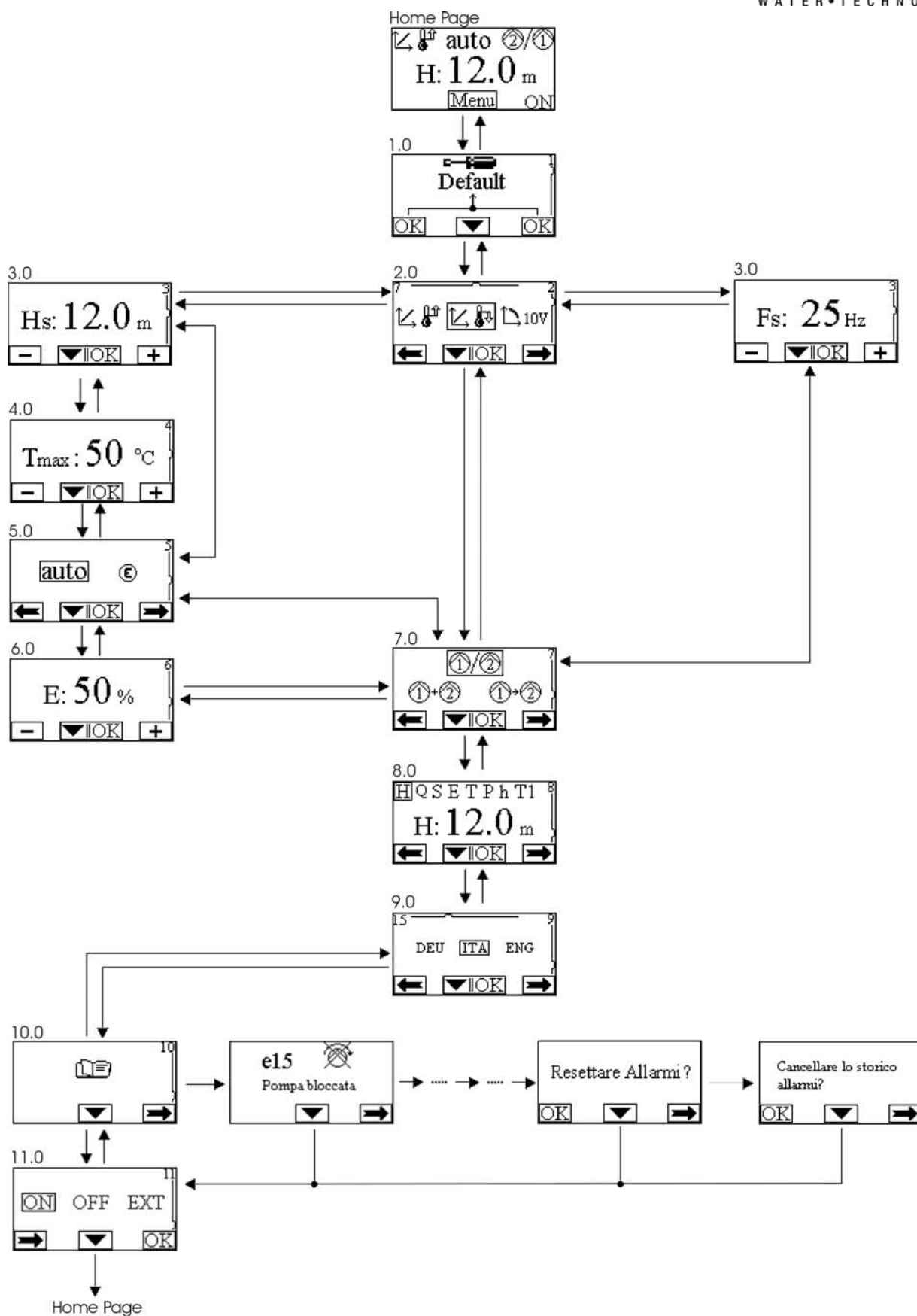
Afbeelding 8: Menu MCE
