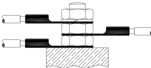
Figura 2: Împământare
