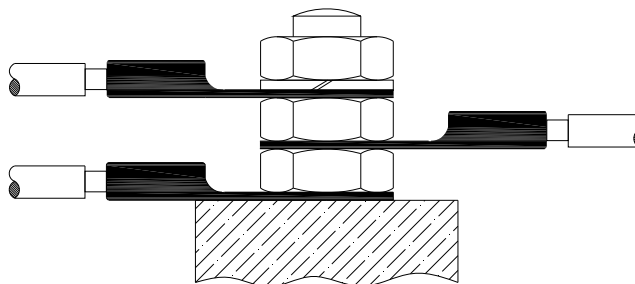
Εικόνα 2: Σύνδεση Γείωσης
