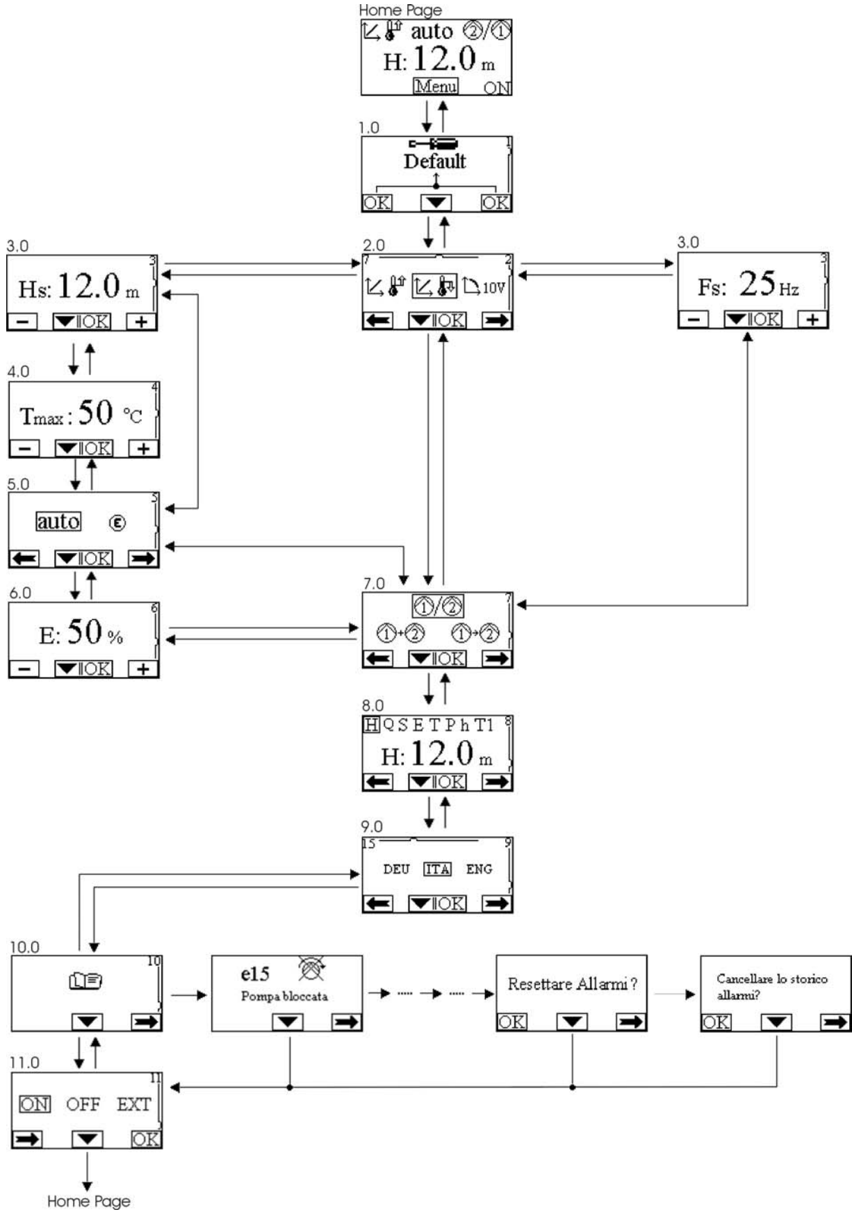
Resim 8: MCE Menüsü
