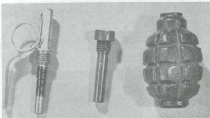
Granada de Mão defensiva, Tipo F-1, origem: Rússia
