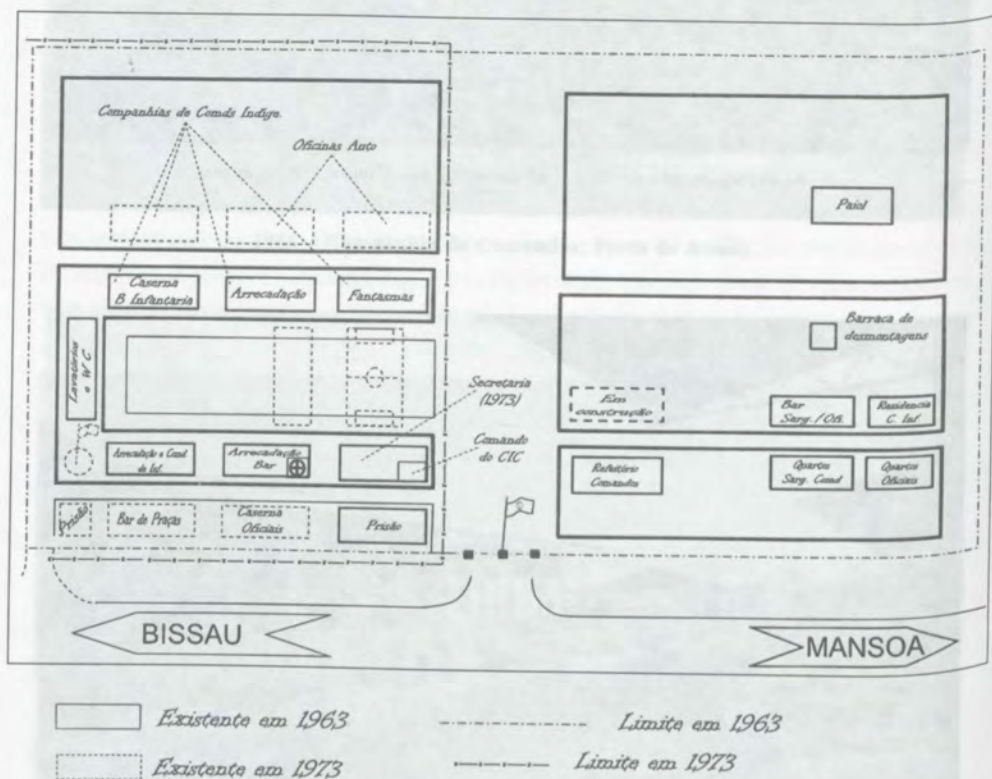
Planta do aquartelamento de Brá – Instalações iniciais e novas áreas edificadas
