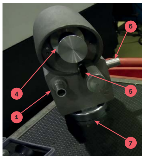
Figura 2. Constituição do Skimmer: 1 – canal de saída da emulsão; 2 – tela polarizada; 3 – roldana inferior; 4 – roldana superior; 5 – raspador; 6 – canal de saída do óleo de guias; 7 – base magnética.
