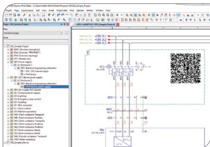
Figura 1 Na plataforma EPLAN, versão 2.9, podem ser gerados códigos QR que, por exemplo, vinculam a um componente na EPLAN Data Portal.
