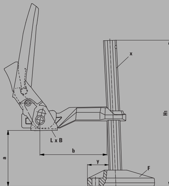
Grampo de aperto com regulação posterior GRS
