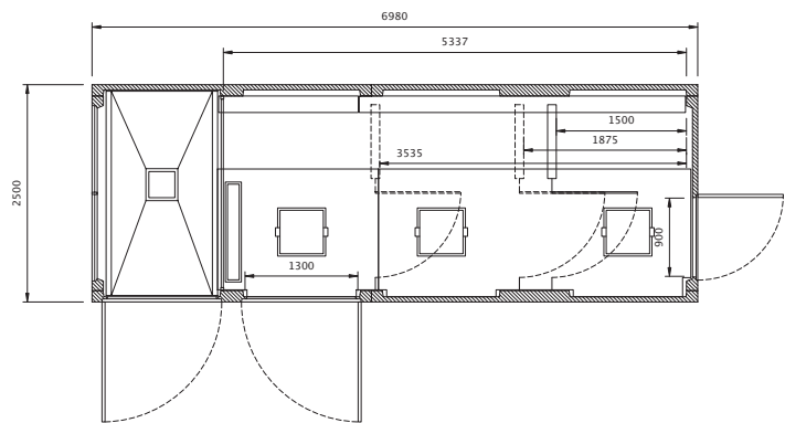
planta EHCP 7 T2E
