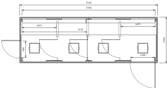
planta EHCP 8 S PL
