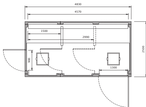
planta EHCP 4 S PL
