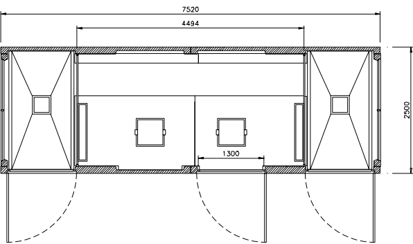
planta EHCP 8 T2L
