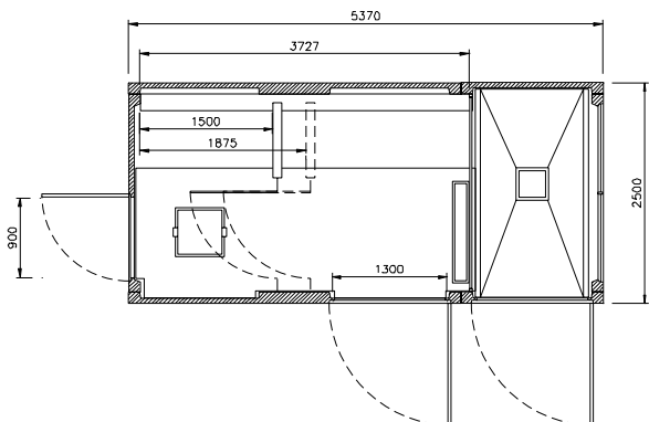
planta EHCP 5 T1D PL
