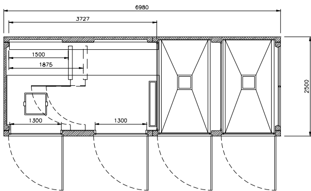
planta EHCP 7 T2E PF
