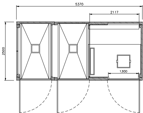
planta EHCP 5 T2E
