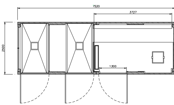
planta EHCP 8 T2E PL
