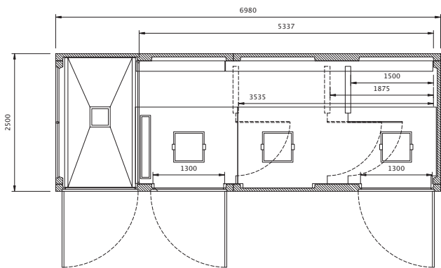
planta EHCP 7 T2D
