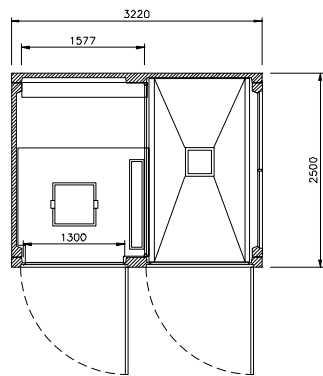
planta EHCP 2 T1D
