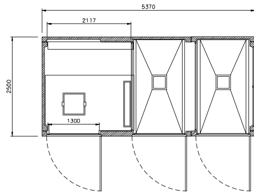
planta EHCP 5 T2D
