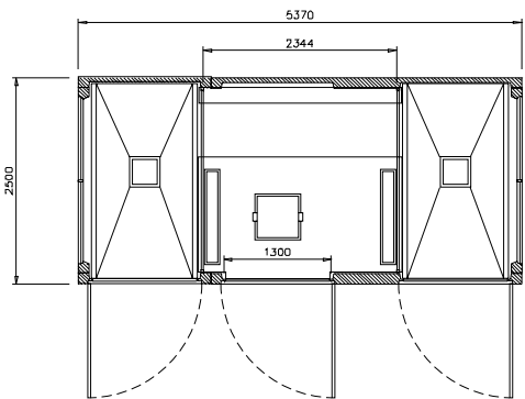
planta EHCP 5 T2E
