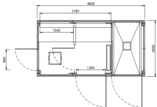
planta EHCP 4 T1D PL
