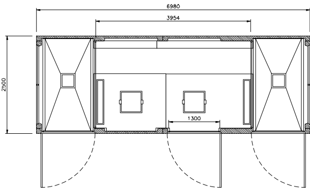
planta EHCP 7 T2L
