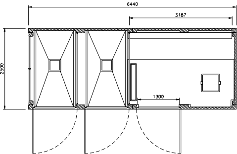
planta EHCP 6 T2E
