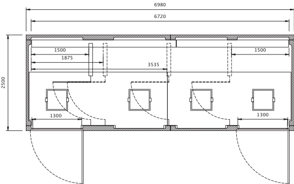
planta EHCP 7 S PF
