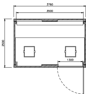
planta EHCP 3 S
