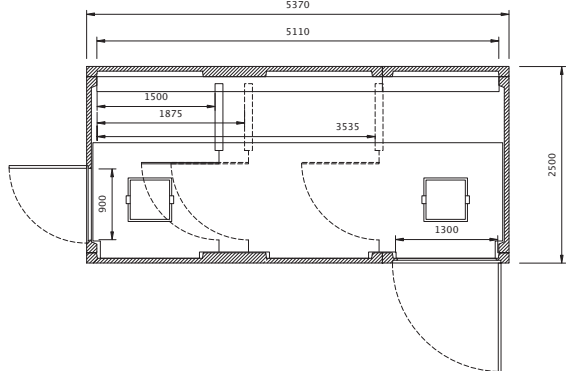
planta EHCP 5 T1E
