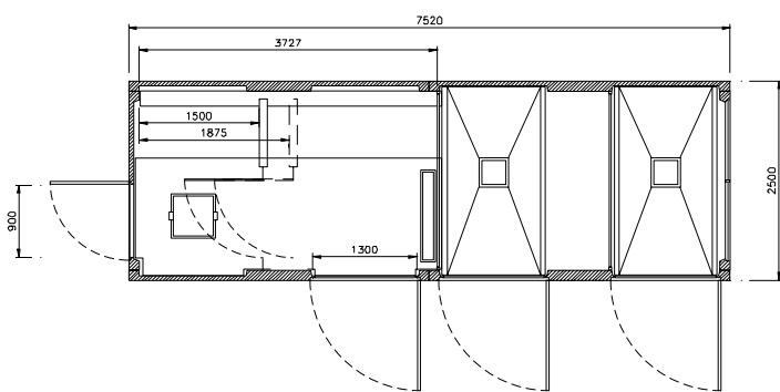
planta EHCP 8 T2E PF
