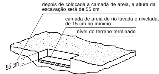
Figura 1 vsta do corte do fosso
