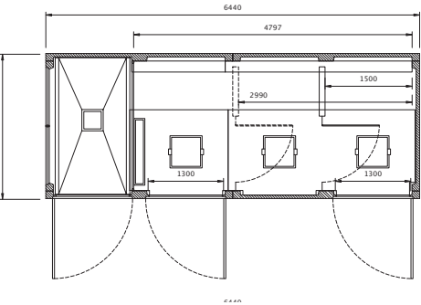
planta EHCP 6 T2D
