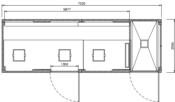
planta EHCP 8 T1D
