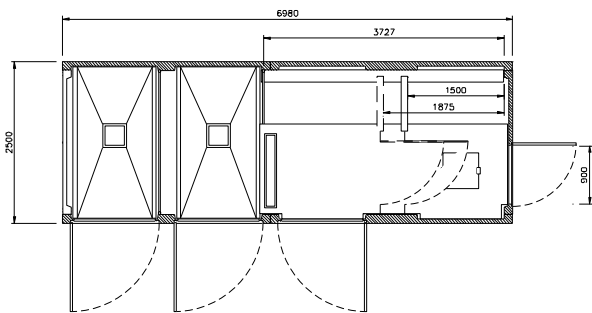
planta EHCP 7 T2E PL
