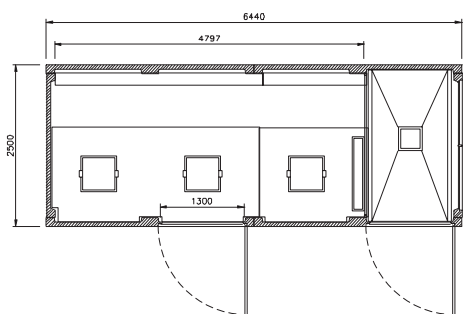
planta EHCP 6 T1D
