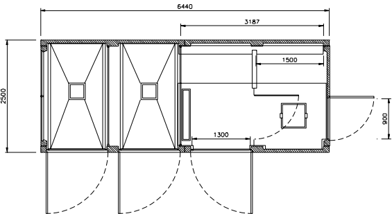
planta EHCP 6 T2E PL
