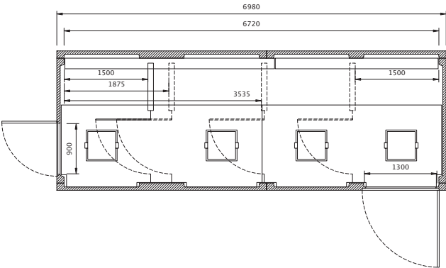
planta EHCP 7 S PL
