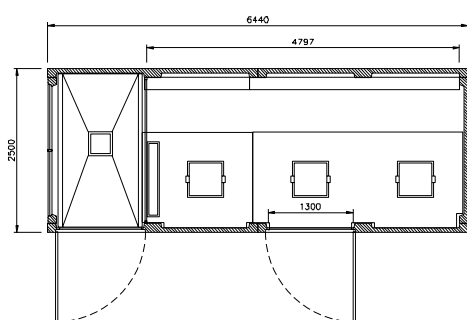
planta EHCP 6 T1E
