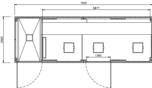
planta EHCP 8 T1E
