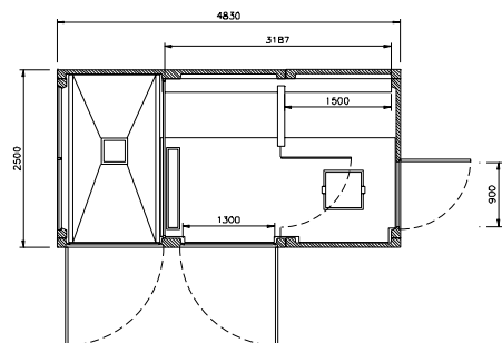
planta EHCP 4 T1E PL
