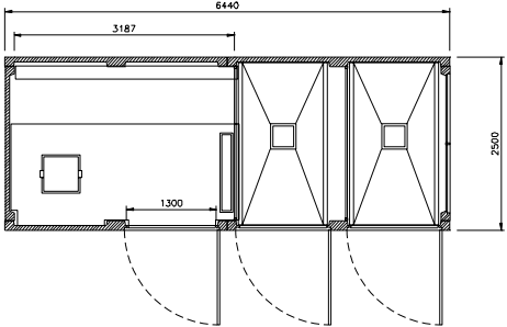
planta EHCP 6 T2D
