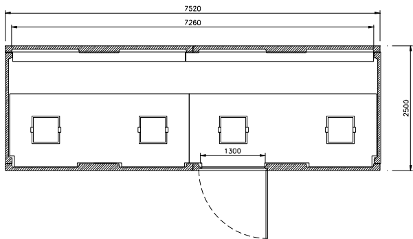
planta EHCP 8 S PL
