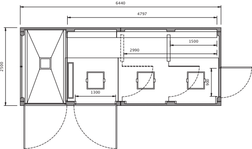
planta EHCP 6 T1E PL
