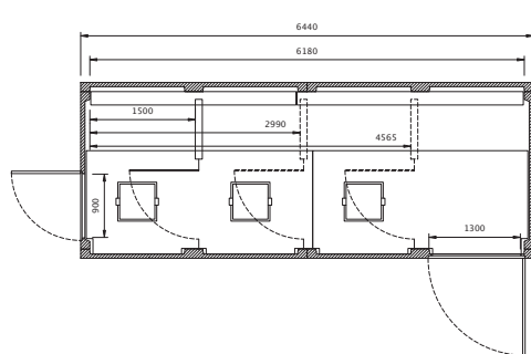
planta EHCP 6 T1E
