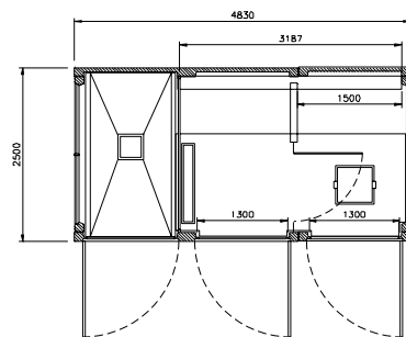
planta EHCP 4 T1E PF
