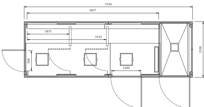
planta EHCP 8 T1D PL
