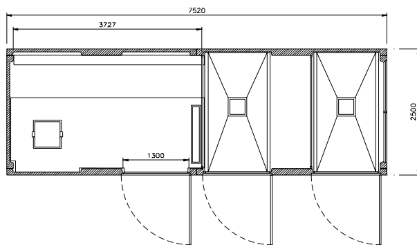
planta EHCP 8 T2D
