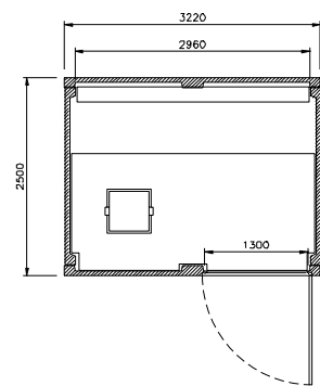
planta EHCP 2 T1E
