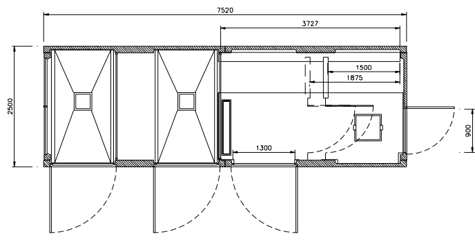
planta EHCP 8 T2E PL
