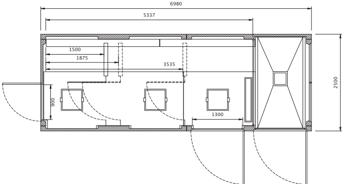
planta EHCP 7 T1D PL
