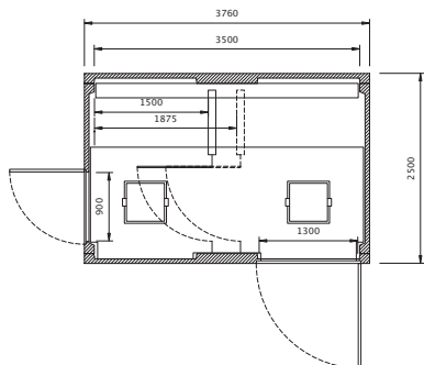
planta EHCP 3 S PL
