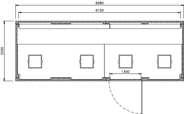
planta EHCP 7 S
