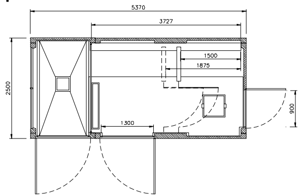
planta EHCP 5 T1E PL
