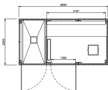
planta EHCP4 T1E
