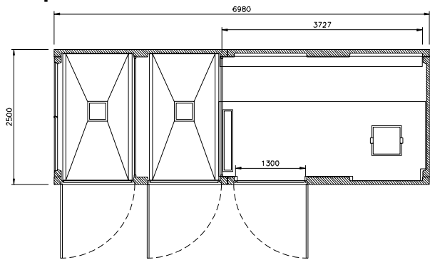
planta EHCP 7 T2E
