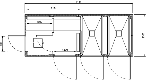
planta EHCP 6 T2D PL
