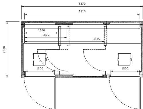
planta EHCP 5 T1D
