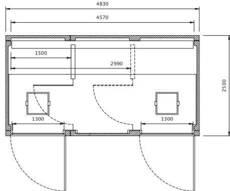
planta EHCP 4 S PL
