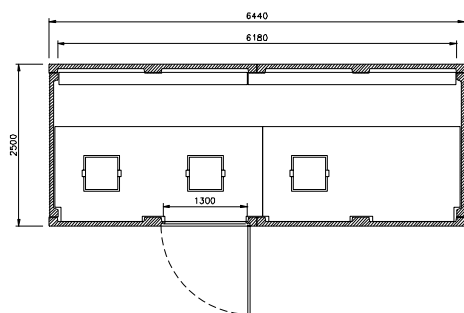
planta EHCP 6 S
