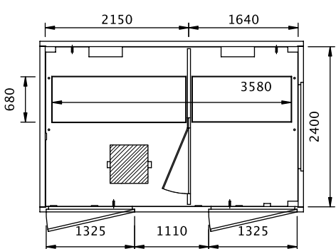
PLANTA M1 S PF 36
