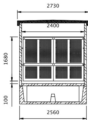
CORTE A-A'
