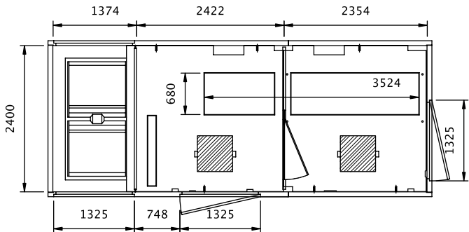
PLANTA M110 T1E PL 36
