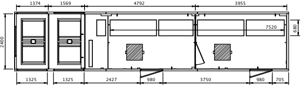
PLANTA M111 T2E PF
