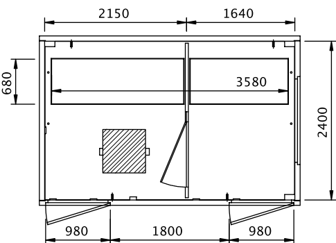
PLANTA M1 S PF
