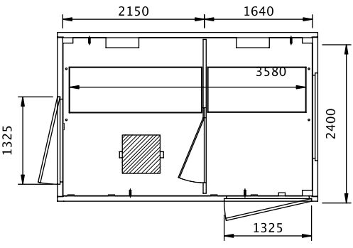
PLANTA M1 S PL 36
