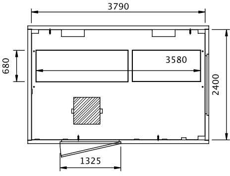
PLANTA M1 S 36
