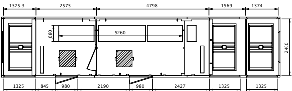
PLANTA M111 T2D1E PF
