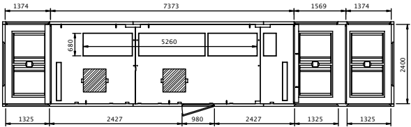
PLANTA M111 T2D1E
