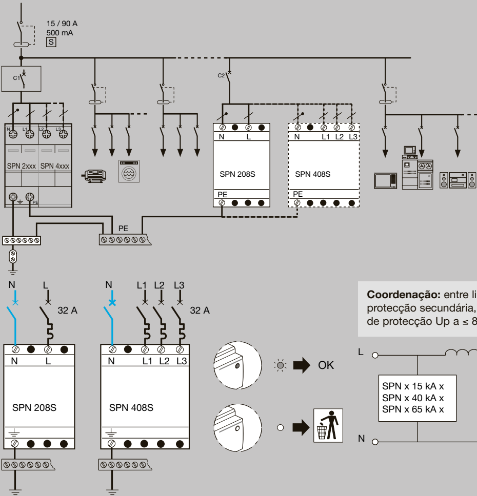
Esquema de princípio de instalação
